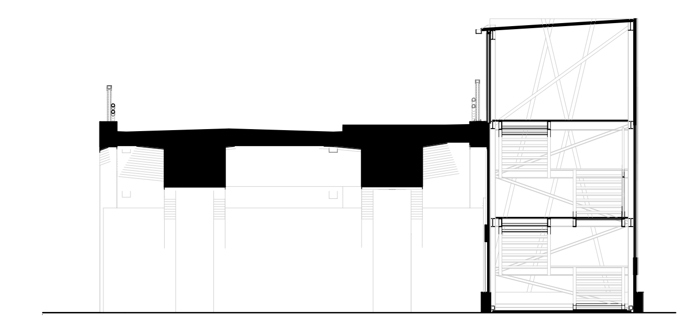
D4 Leikkaus D-D 1:100
