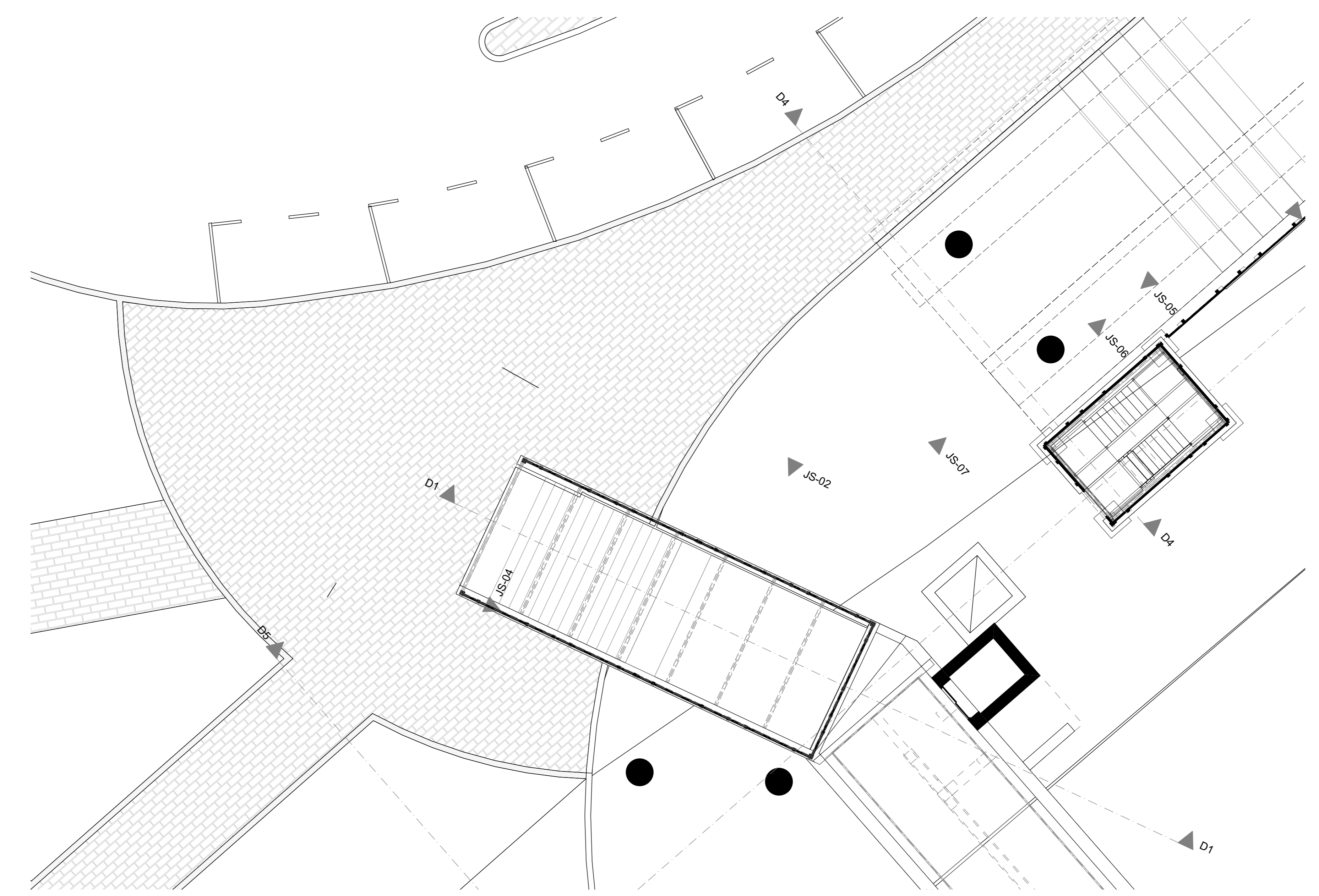
5. 27.10 LAITURI (+25.000) 1:100
