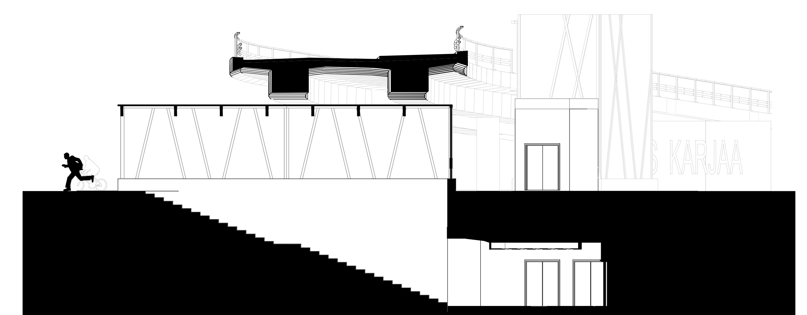
D1 Leikkaus D-D 1:100
